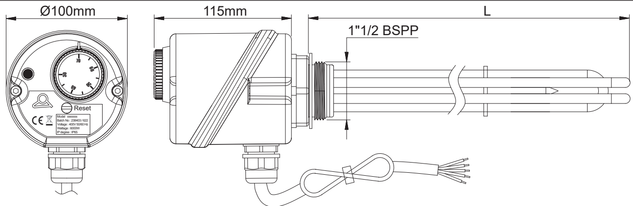
3-poliger 400V-Heizer
