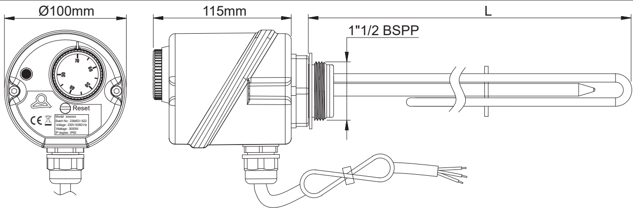
1-poliger 230V-Heizer
